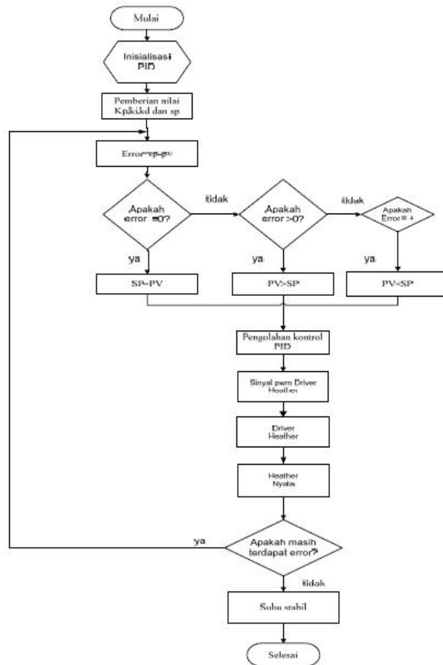
Gambar 3. Diagram alir program utama
